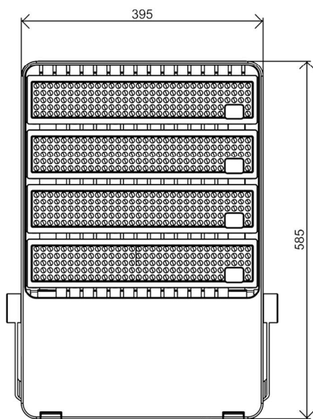
主视图
